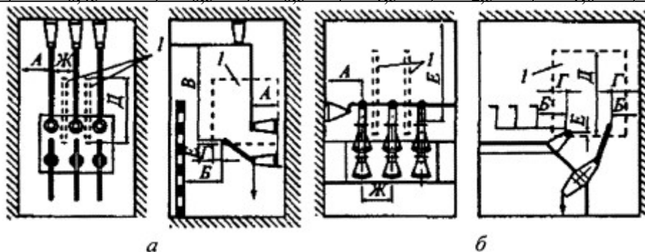
Рис. 4.2.2. Установка разъединителя (отделителя): а
