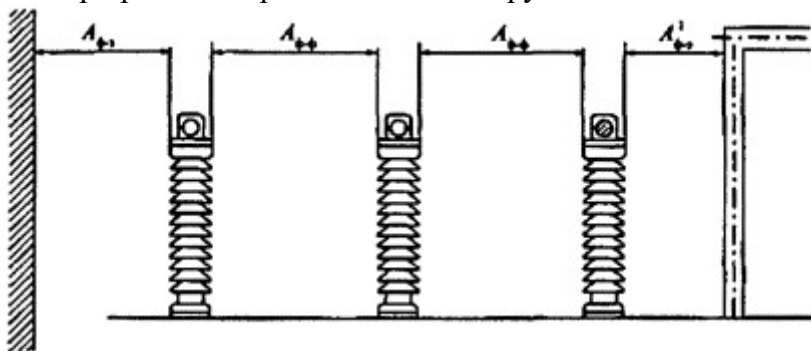
Рис. 4.2.3. Наименьшие расстояния в свету при жестких шинах между токоведущими и
